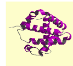
1hbbA0
