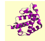
1hbbB0
