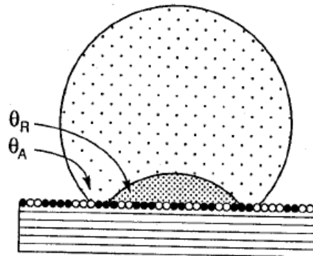
Ετερογένεια
