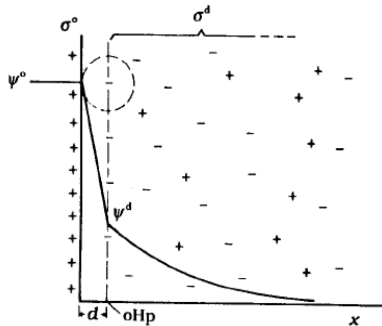
Μοντέλο Gouy-Stern
